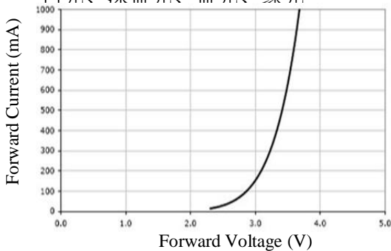
5-1. White, Royal Blue, Blue, Green 白光、深蓝光、蓝光、绿光
