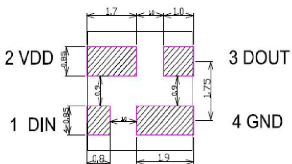
背部建议焊盘尺寸
