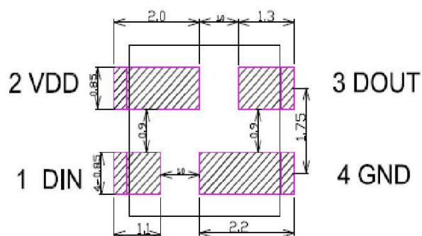
背部建议钢网尺寸
