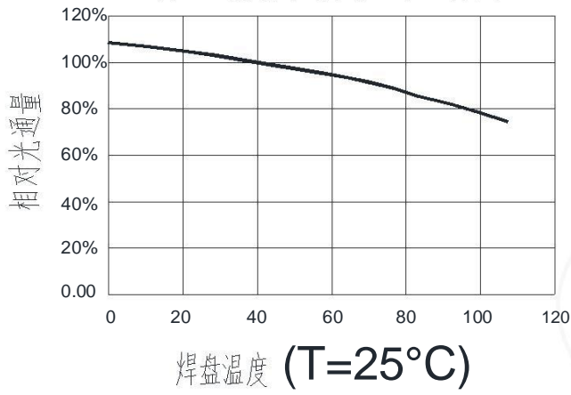
焊盘温度与光通量输出的相对关系
