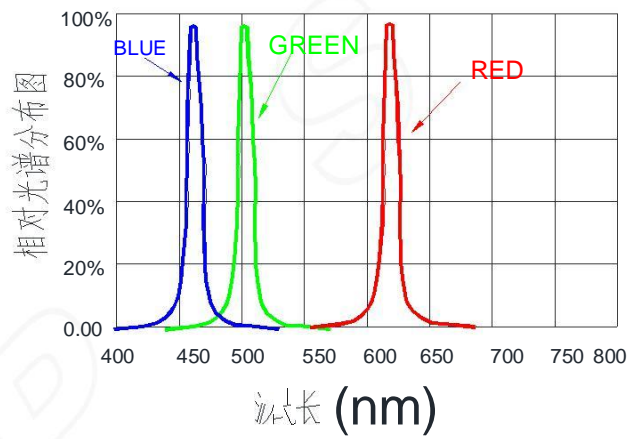
波长特性
